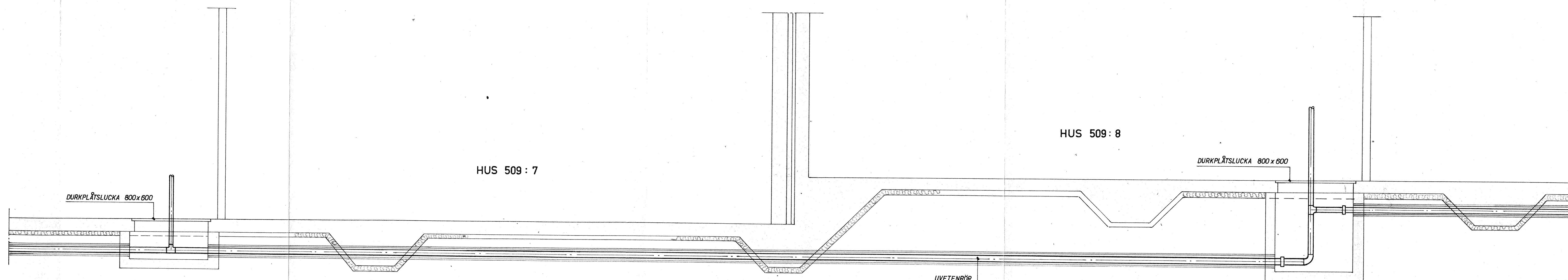
SEKTION GÄLLER HUS 509:7-:8 SKALA 1:20
