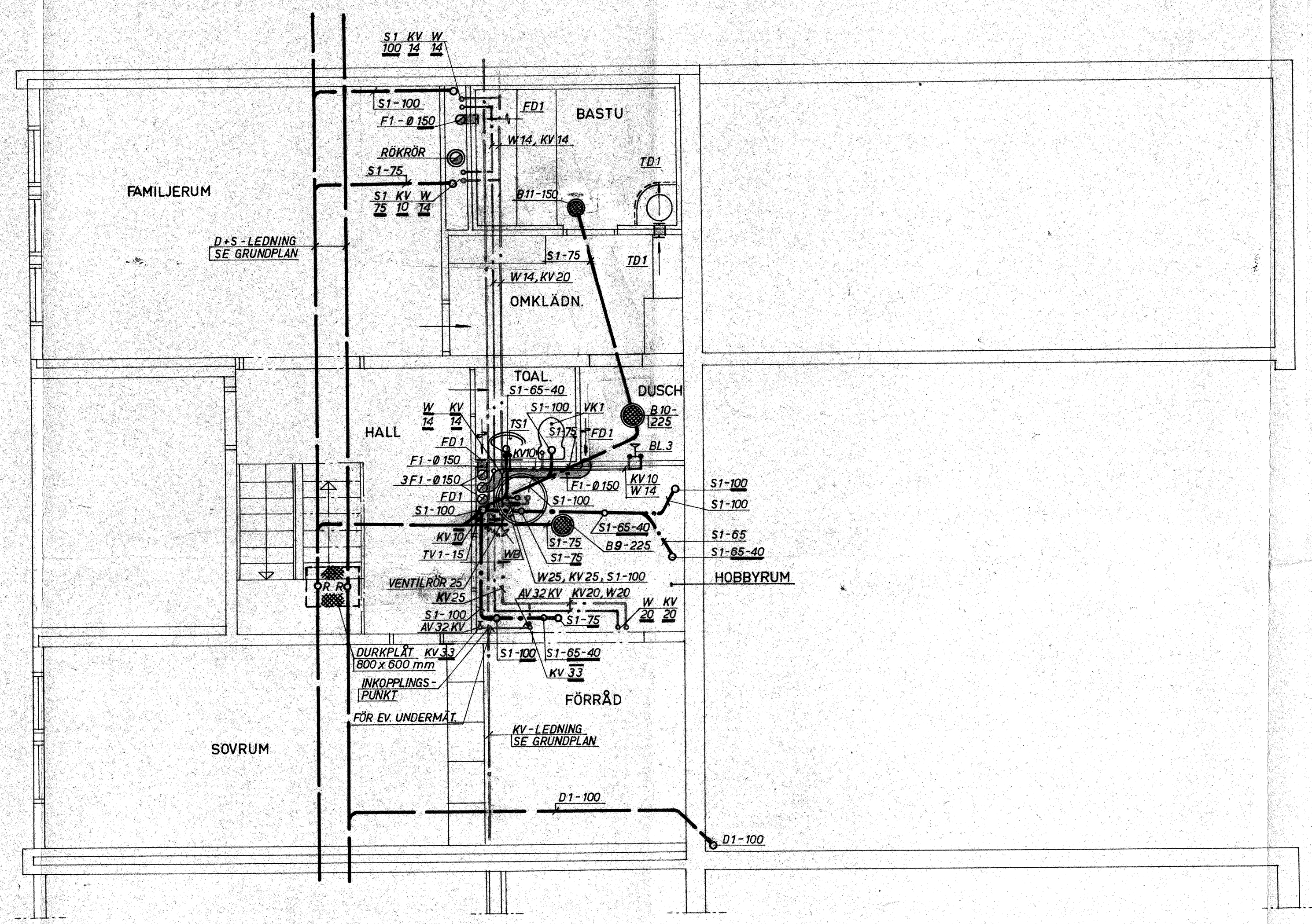
SOUTERRÄNGPLAN
