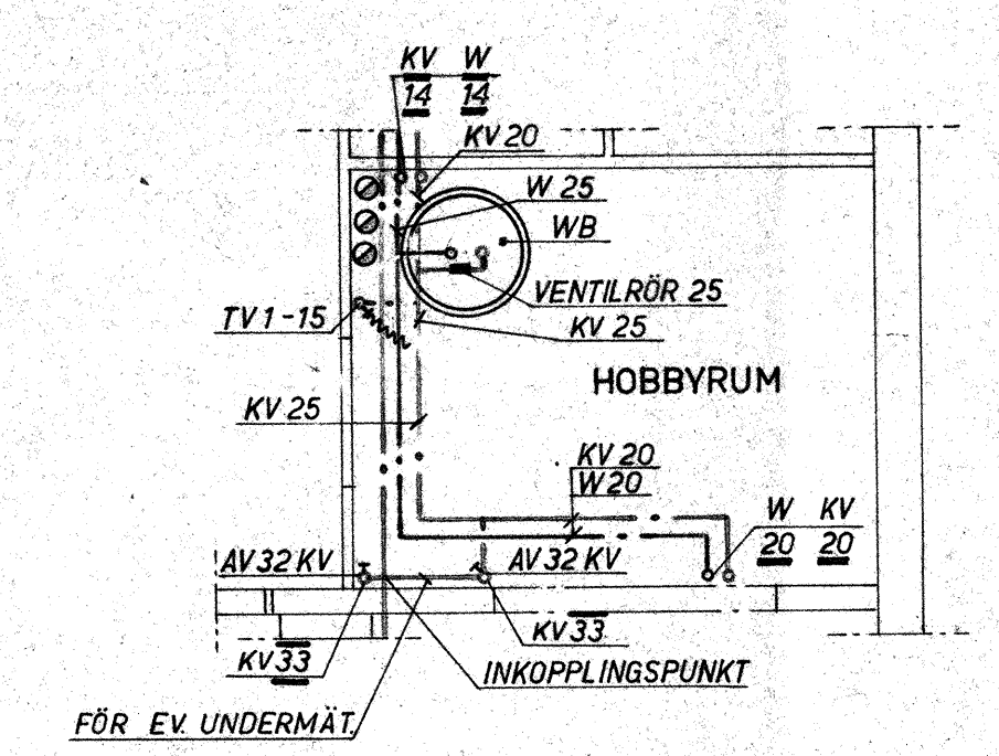
SOUTERRÄNGPLAN
