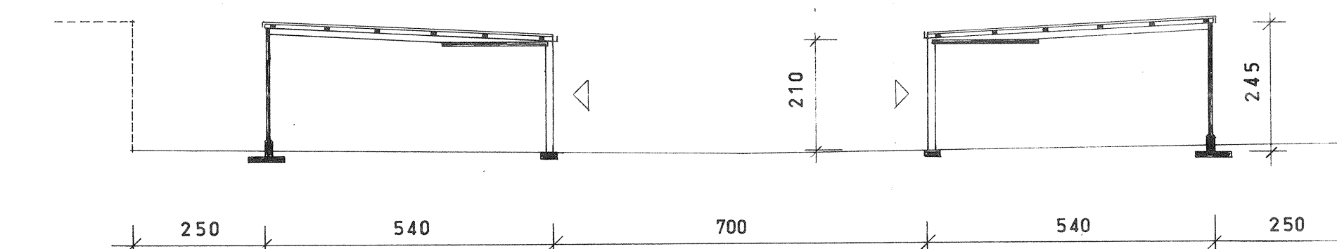
SEKTION
