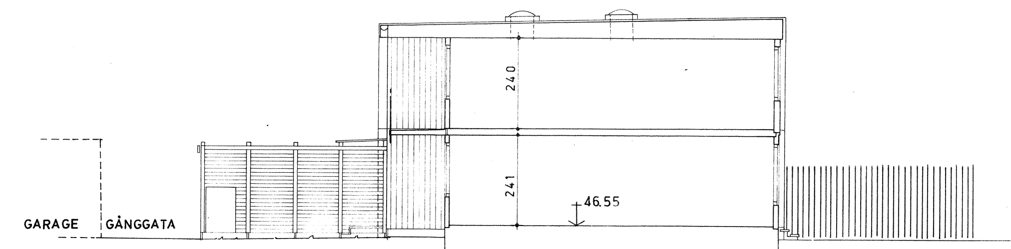
SEKTION
